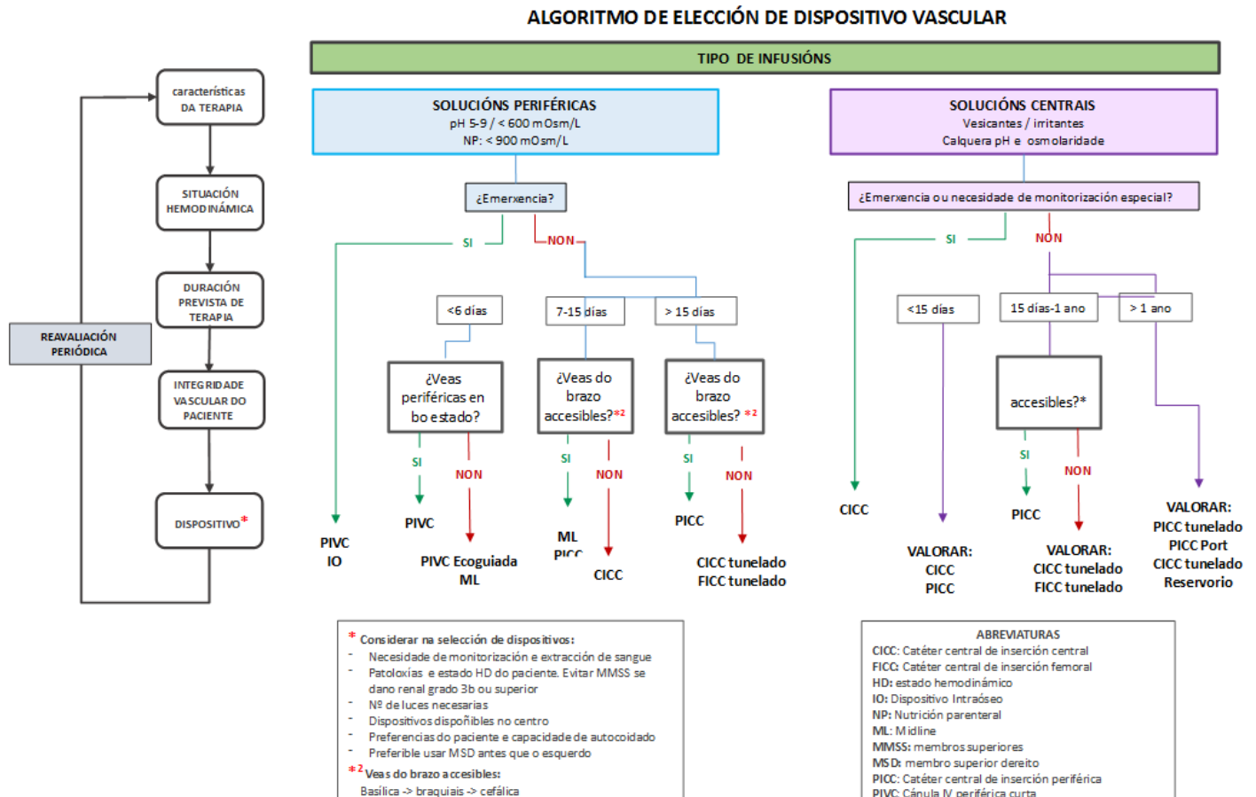
FIGURA 1 ALGORITMO 1,2,3
